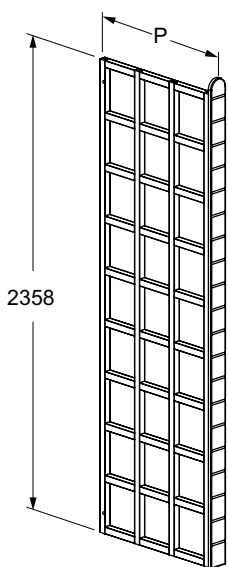
291 - Боковина решётчатая левая.
